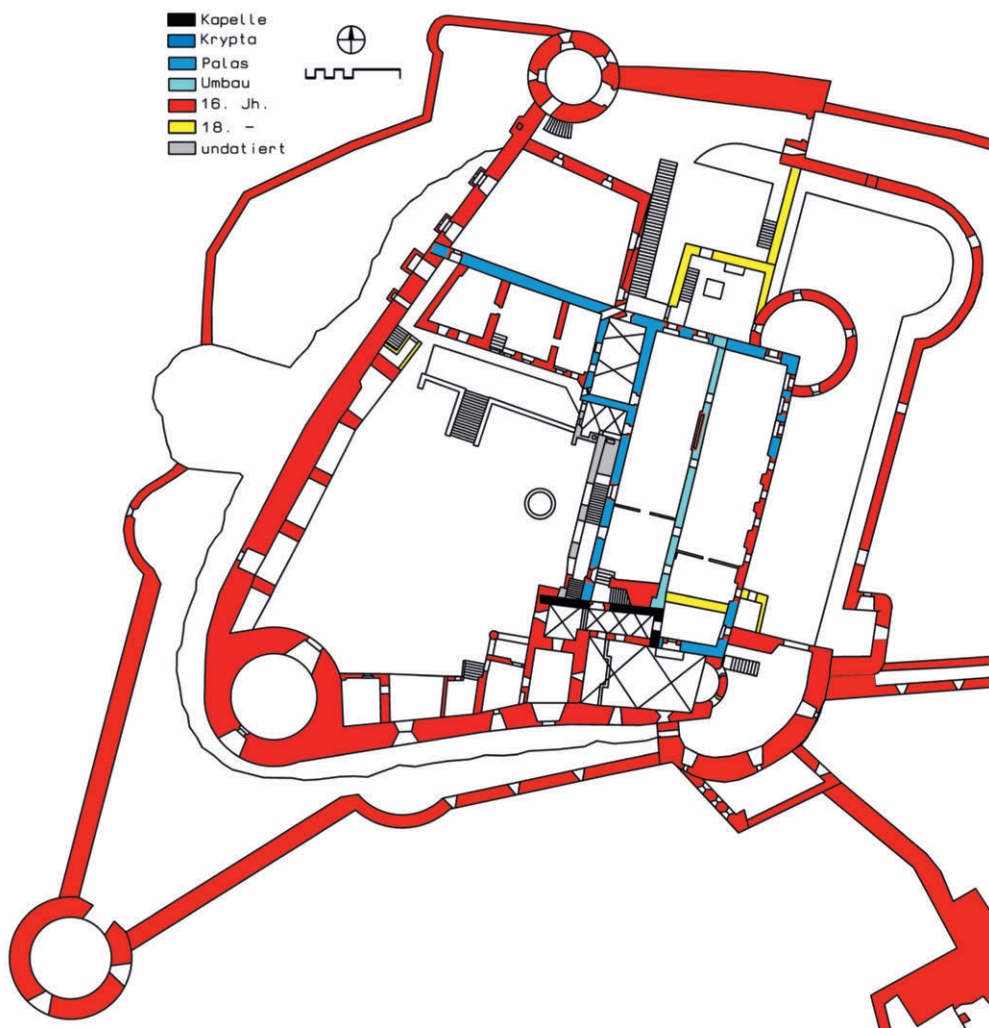
Kernburg Hohenwerfen, Baualtersplan der Kernburg
