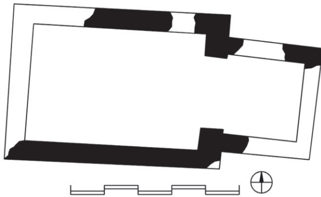
Wildon, Grundriss der Burgkapelle
