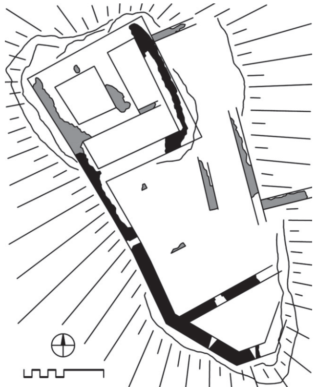
Stall-Wildegg im Mölltal, Gesamtanlage, schwarz: ältere Teile
