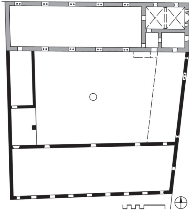
Salzburger Hof in Regensburg, 1. Obergeschoß, Phasen bis ins mittlere 13. Jahrhundert, grau: älter
