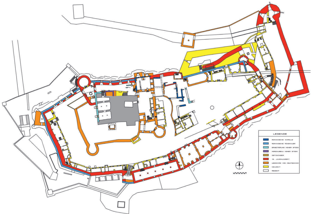
Festung Hohensalzburg, Baualtersplan des Hauptniveaus
