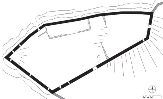
Plainburg, Kernburg, schwarz: ältere Teile
