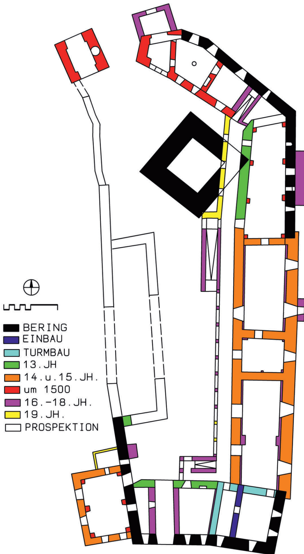
Kernburg Seggau, Baualtersplan des Hofniveaus
