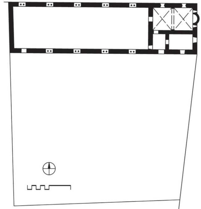
Regensburg, Salzburger Hof, Rekonstruktion des 1. Obergeschoßes unter Konrad III.
