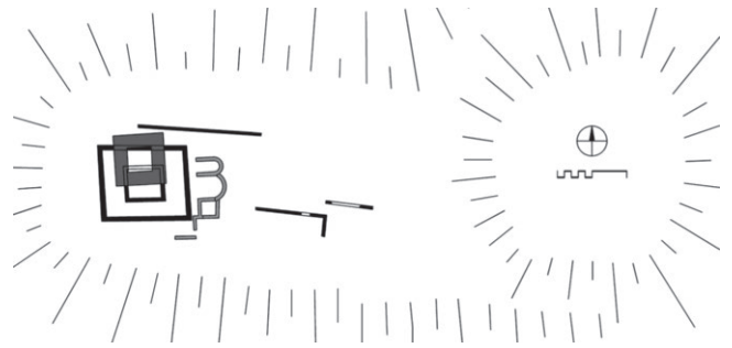
Pettau/Ptuj, Grabungsergebnisse: vermutlicher kaiserzeitlicher Umgangstempel mit Terrassenmauern, vermutlicher spätrömischer Turm bzw. Burgus (starke Mauern) und wohl direkt angestellte Ostpartie einer Kirche. Östlich mag Salzburg auf dem eigentlichen Gipfelplateau eine Burg errichtet haben, die archäologisch nicht erforscht ist
