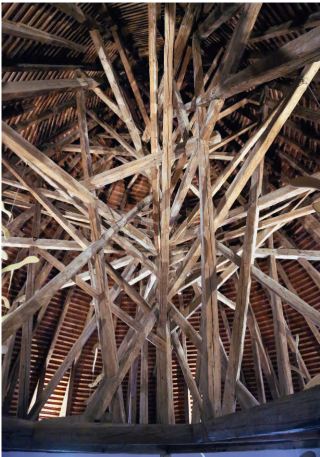
Reichenburg/Rajhenburg, Dachkonstruktion des runden Flankenturms
