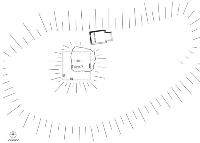
Hohensalzburg, erhaltene Bauten bis zum späten 11. Jahrhundert
