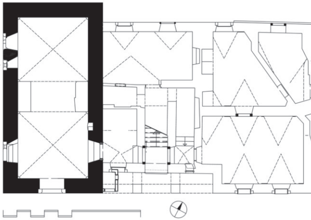
Rüstenau/Ristovec bei Pettau/Ptuj, Grundriss des Erdgeschoßes mit Hervorhebung des Kernbaus
