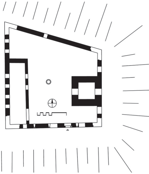
Liechtenwald/Sevnica, Grundriss 1. und 2. Bauphase
