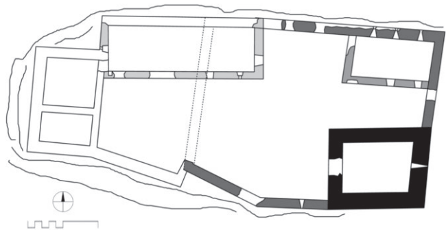
Kaprun, romanische Bauphasen
