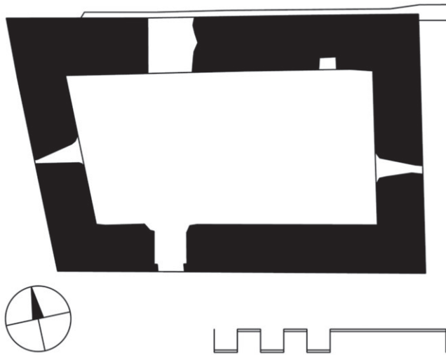
Megling, Erdgeschoß des Festen Hauses
