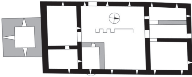
Hörberg/Podsreda, romanische Bauphasen der Kernburg, schwarz: älteste Teile
