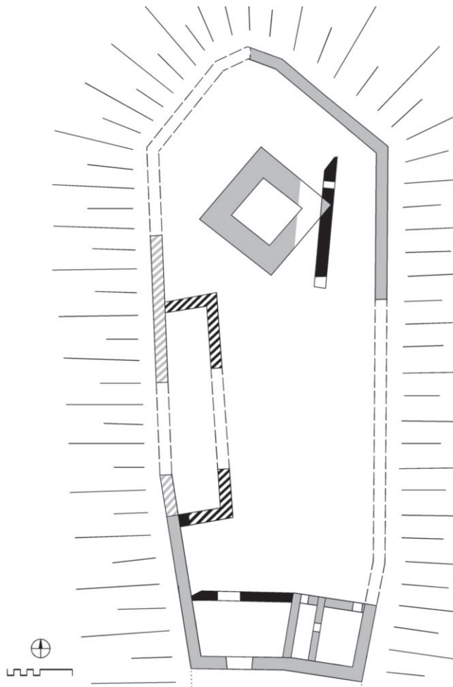
Leibnitz, vermutliche Bauten bis zum mittleren 13. Jahrhundert, grau: älter
