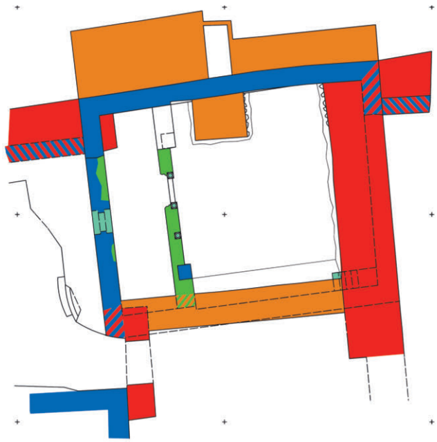
Festung Hohensalzburg, Baualtersplan des Hohen Stocks im ausgegrabenen Untergeschoß
