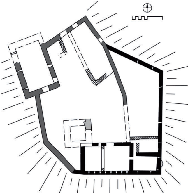
Reichenburg, Bauphasen des 12. Jahrhunderts, schwarz: Konrad III.
