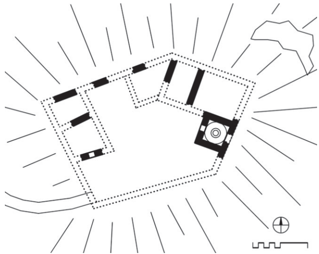
Reichenstein/Reštanj, Grundriss
