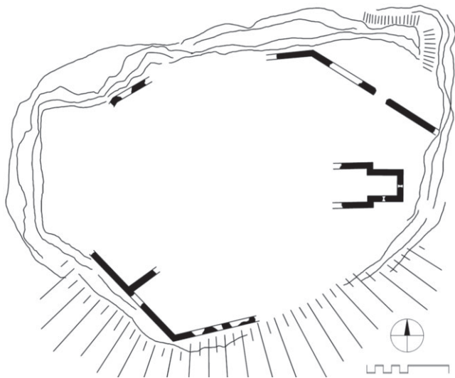
Karlstein, Kernanlage, Bauten des 12. Jahrhunderts
