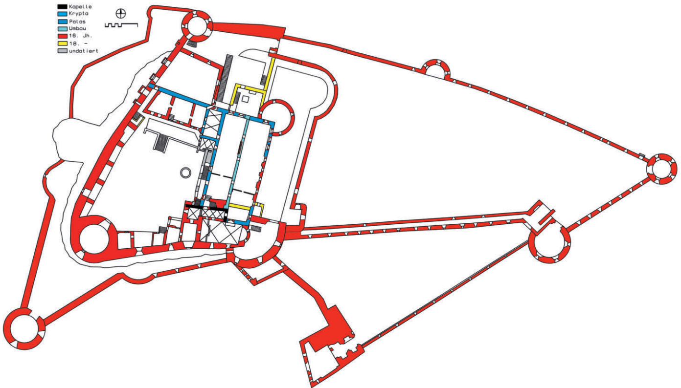
Hohenwerfen, Baualtersplan der Gesamtanlage
