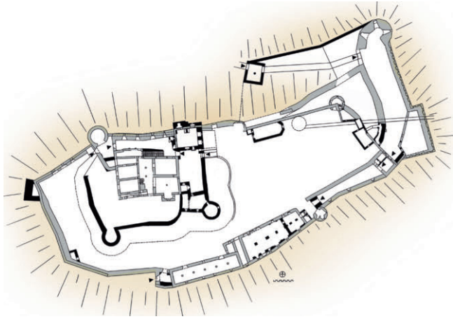
Hohensalzburg, Baumaßnahmen unter Erzbischof Leonhard, grau: älter
