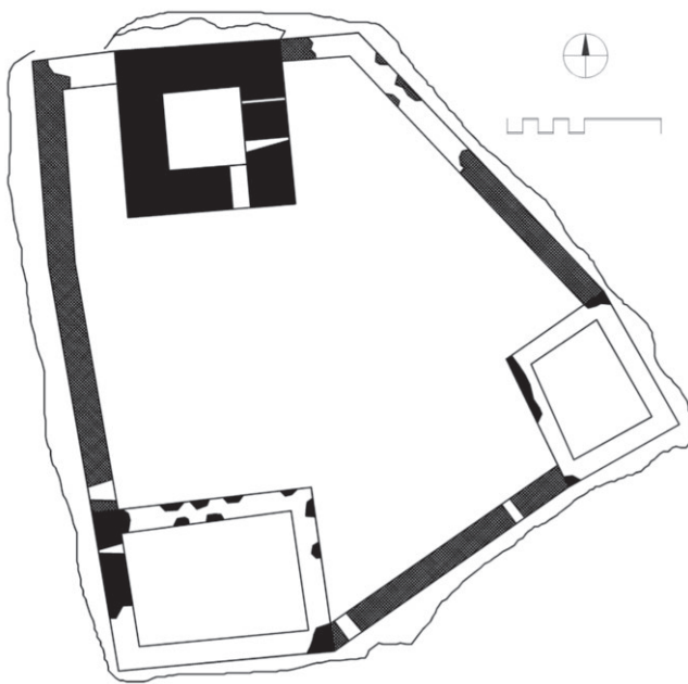
Hieburg, Bauphasen des 13. Jahrhunderts
