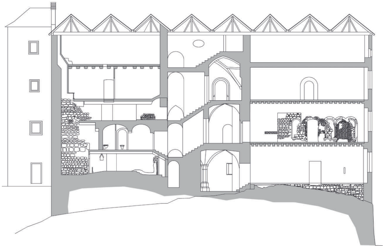
Festung Hohensalzburg, Querschnitt durch den Hohen Stock von West nach Ost in Richtung Nord entlang der Südfassade mit Eintragung bekannter Baubefunde
