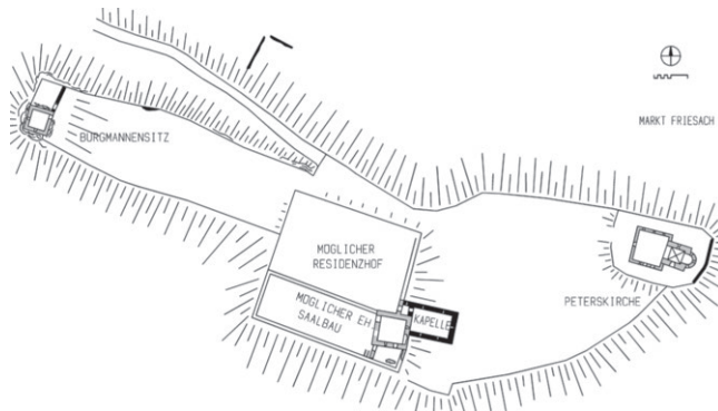
Friesach, Petersberg, Baustufen bis um 1200, schwarz: jüngste Phasen
