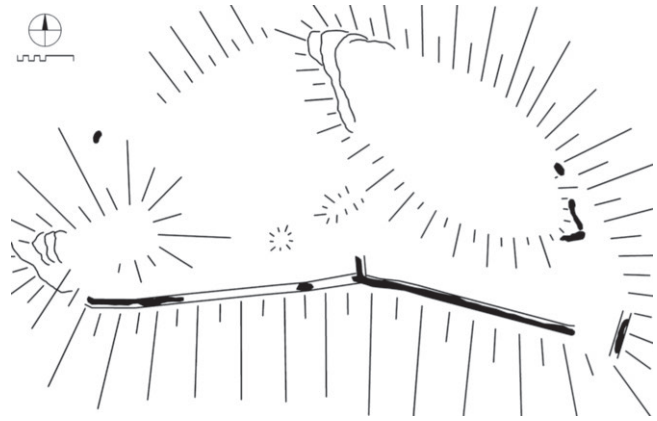
Kirchberg, Gesamtanlage
