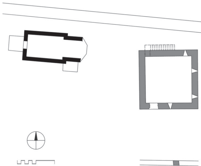
Felberturm, Übersichtsplan
