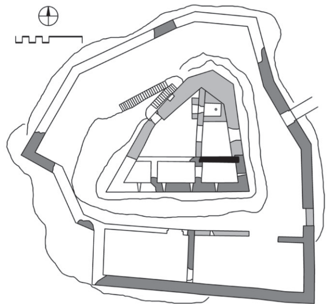
Stein im Lavanttal, romanische Bauphasen, schwarz: älteste Teile
