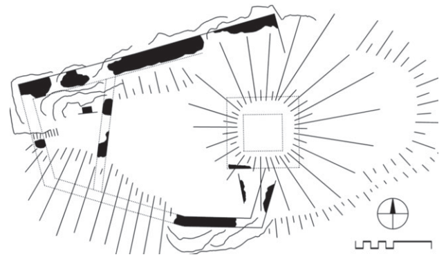
Statteneck, Gesamtplan
