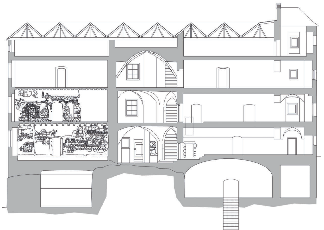
Festung Hohensalzburg, Querschnitt durch den Hohen Stock von Ost nach West in Richtung Süd durch den Kernbau mit Eintragung bekannter Baubefunde
