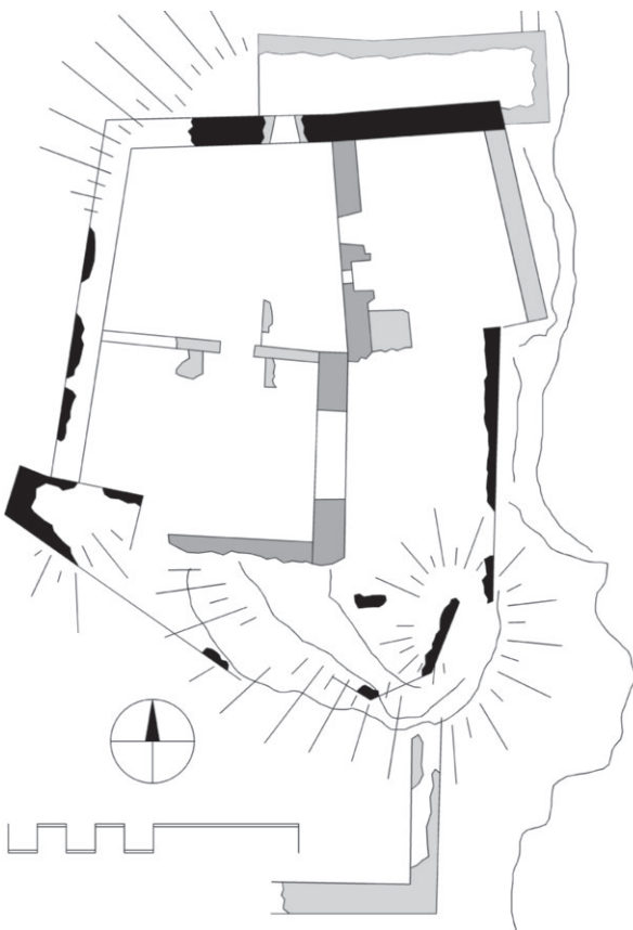
Leobenegg, Gesamtanlage, schwarz: älteste Teile
