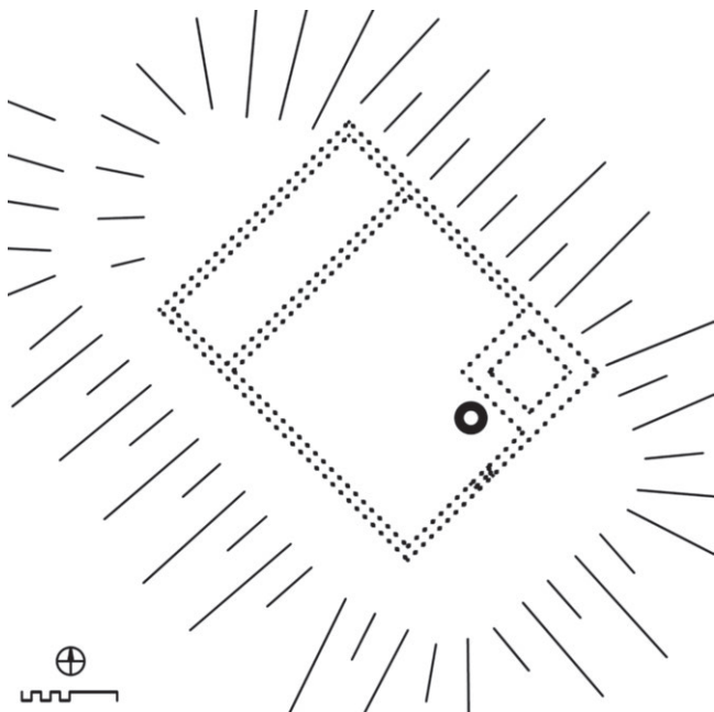
Lutzenwerde, Rekonstruktionsversuch der 1. Bauphase
