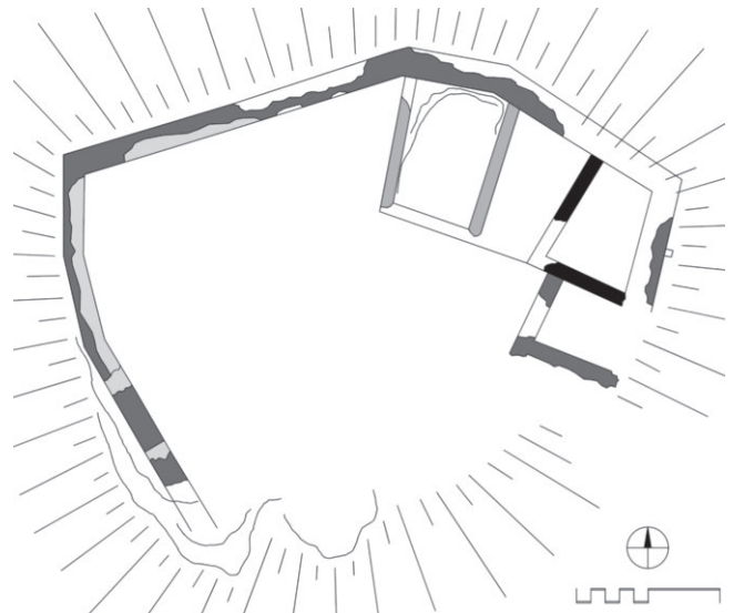
Feldsberg, Kernburg, schwarz: älteste Teile
