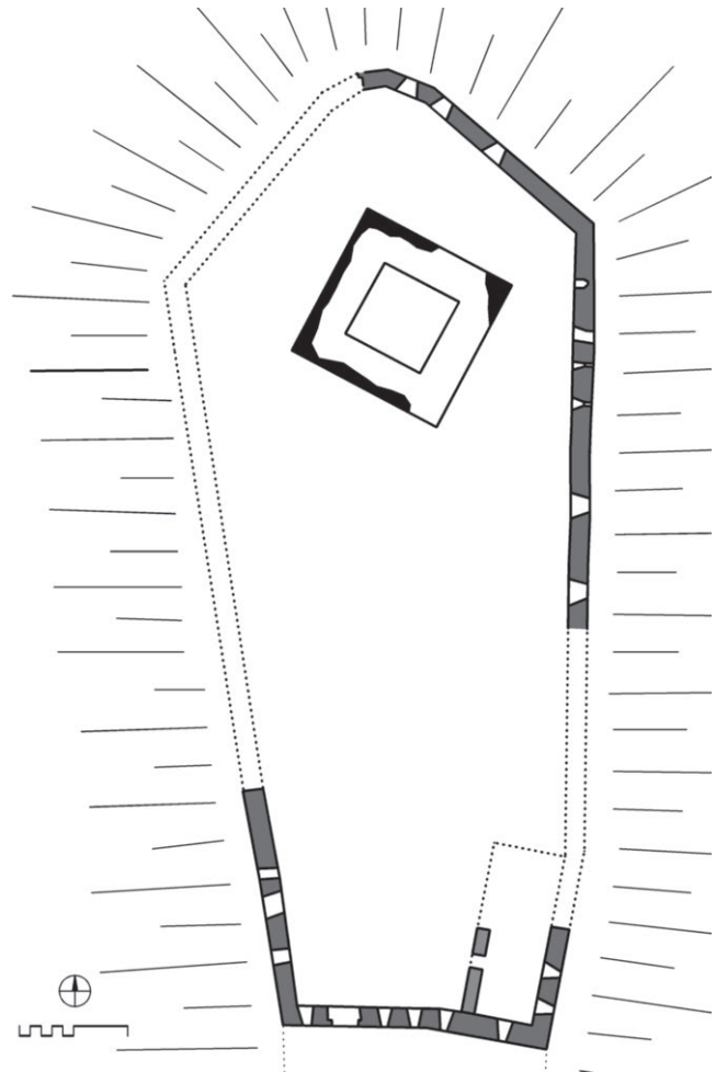
Seggau, Bauten bis Mitte 12. Jahrhundert, schwarz: älter
