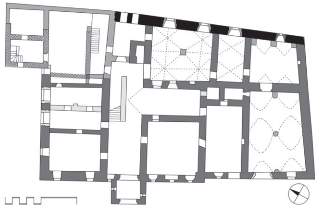
Werfen, Altes Pflegergericht. Schwarz: wohl Hochmittelalter, schraffiert: Mitte 15. Jahrhundert, dunkelgrau: um 1483
