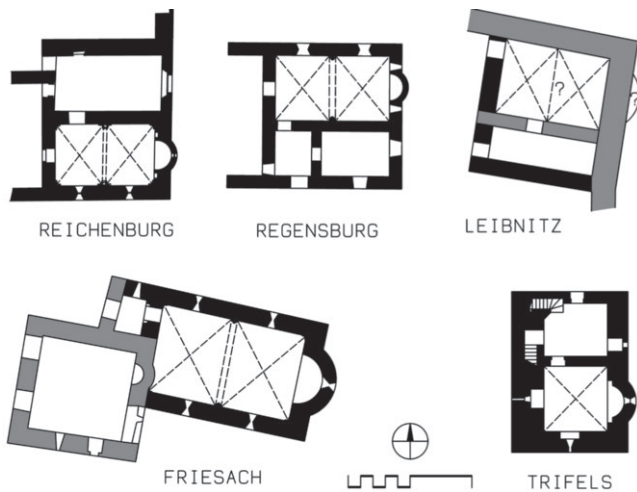
Kapellentürme mit auskragender Apsis an Salzburger Burgen sowie am kaiserlichen Trifels, grau: älter
