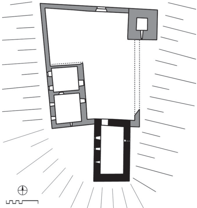
Friedau/Ormož, Grundriss der 1. und 2. Bauphase
