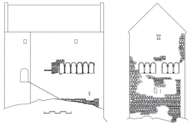
Hohensalzburg, Rekonstruktion des Hohen Stocks mit Kartierung freiliegender Mauerstrukturen
