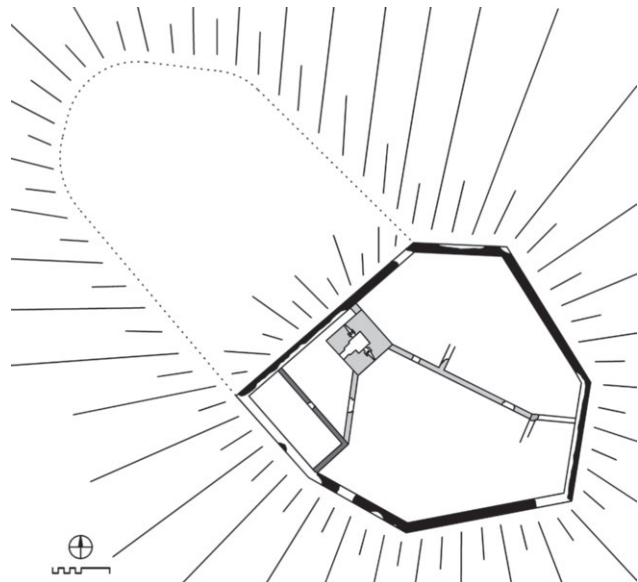
Sachsenburg, Gesamtplan der Mittelburg, grau: später
