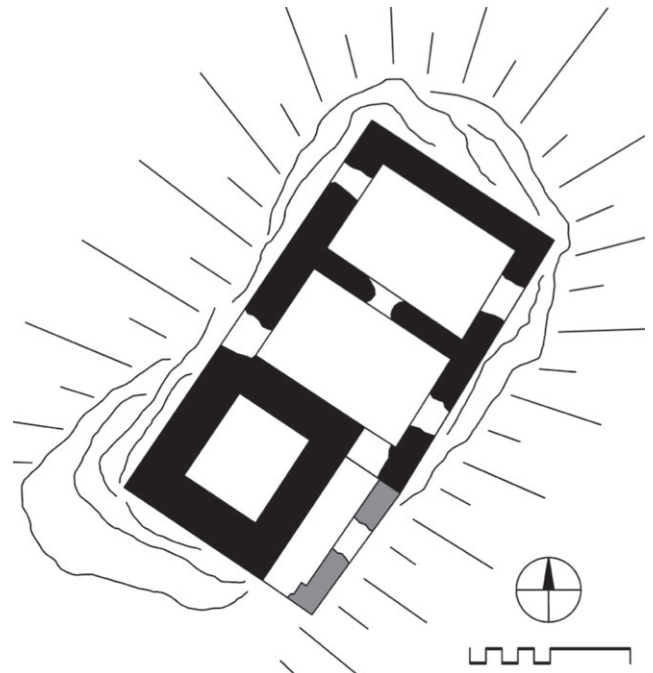
Waxenegg, Bauphasen der Kernburg bis zum mittleren 13. Jahrhundert, schwarz: älteste Phase
