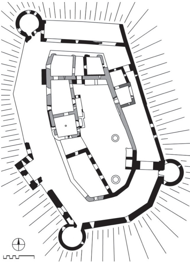
Taggenbrunn, schwarz: spätgotische Ausbauten
