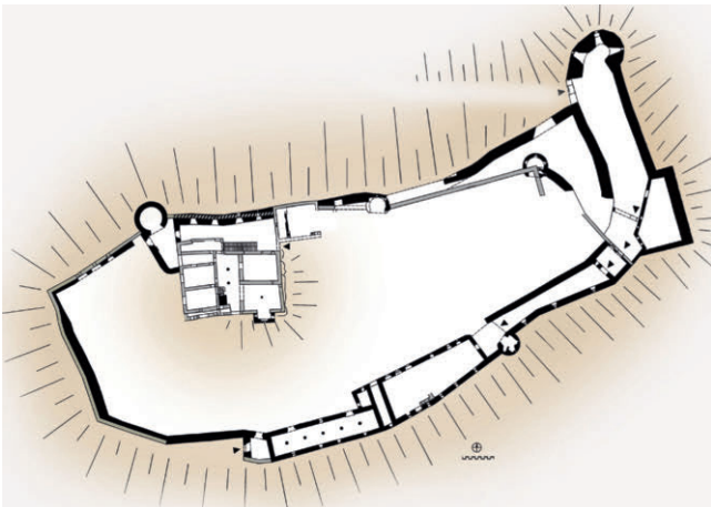
Hohensalzburg, schwarz: Ausbauten im 2. Drittel des 15. Jahrhunderts
