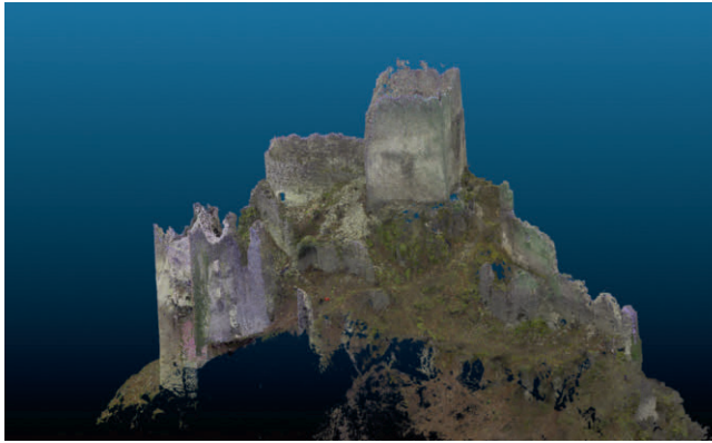
Digitales Modell der Ruine der Gurker Burg Königsberg/Kunšperk, erstellt 2025 auf Grundlage einer 3D-Laserscan-Vermessung vor Ort
