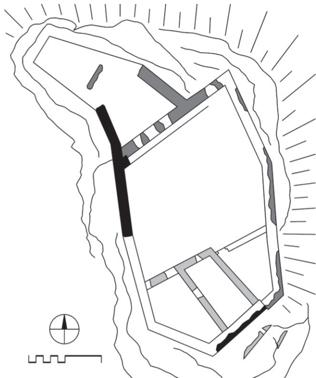
Kienburg in Osttirol, Bauphasen des 12. und 13. Jahrhunderts, schwarz: älteste Teile
