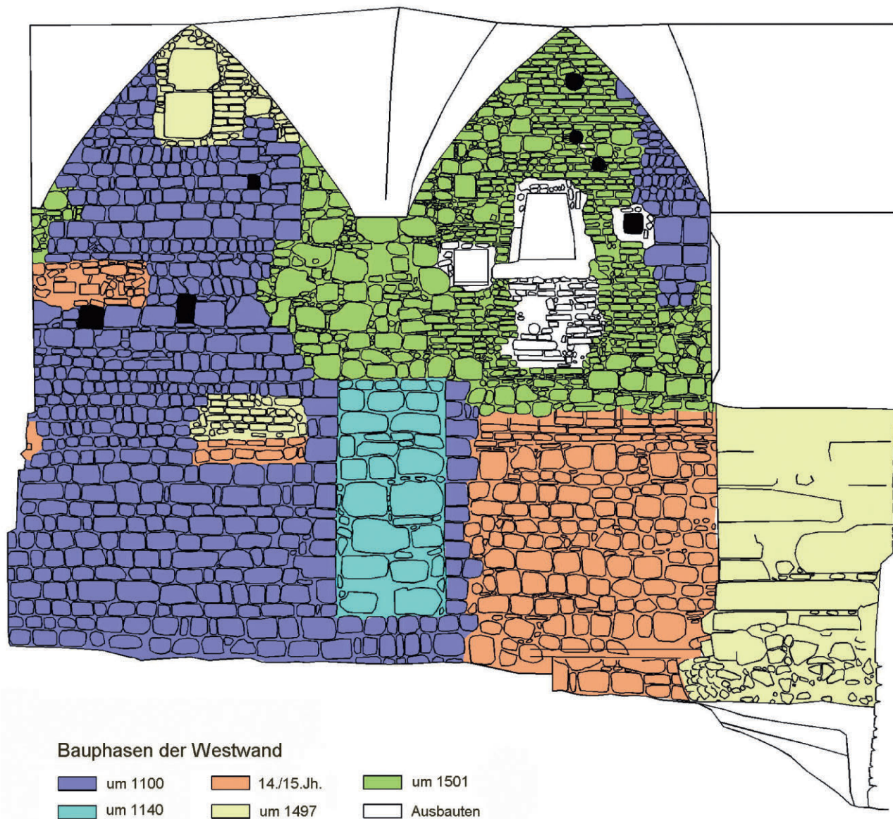
Festung Hohensalzburg, Baualtersanalyse der Westwand der Romanischen Kapelle von innen aus gesehen
