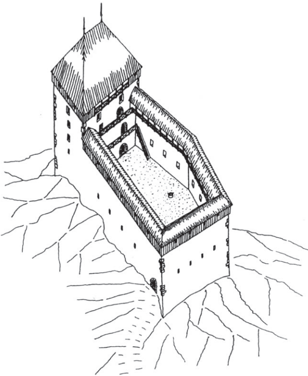
Wurmberg/Vurberk, Hypothetische Rekonstruktion der Erstphase
