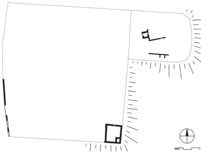
St. Andrä im Lavanttal, Bauteile der 1. Hälfte des 13. Jahrhunderts
