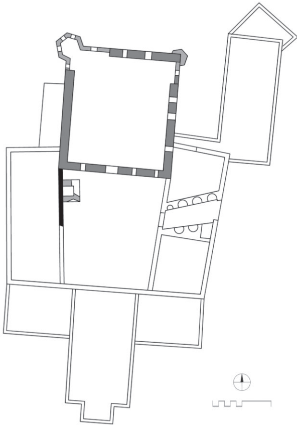
Elsbethen, Schloss Goldenstein, Bauphasenplan
