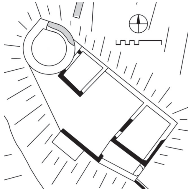
Friesach, Burg Lavant im mittleren 13. Jahrhundert, grau: älter
