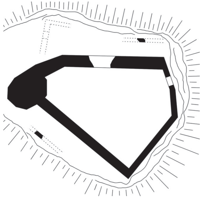
Thurnschall, Gesamtanlage
