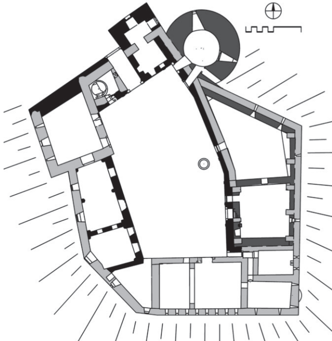
Reichenburg/Rajhenburg, spätgotische Ausbauten, grau: älter
