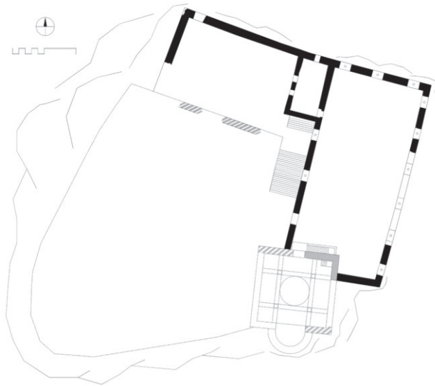
Hohenwerfen, Hauptgeschoß der Kernburg unter Konrad I., grau: älter
