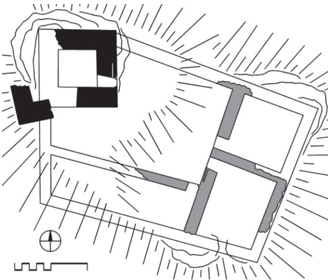
Fohnsdorf, Gesamtplan, schwarz: älterer Turm
