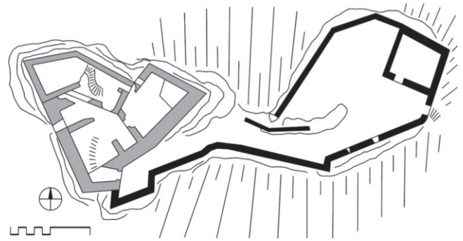
Wartenfels, Gesamtplan, grau: älter
