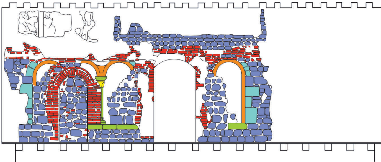
Festung Hohensalzburg, Materialanalyse der südlichen romanischen Fensterarkade im Hohenstock von innen aus gesehen
