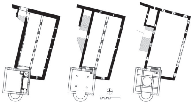
Hohenwerfen, die drei Geschoße des Saalbaus neben der älteren Kapelle
