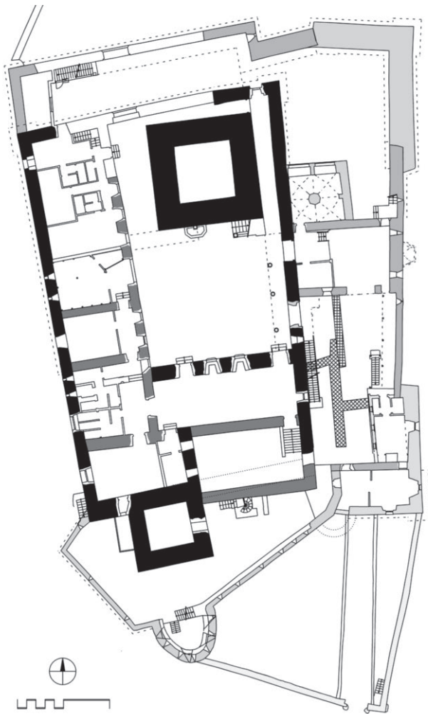
Mauterndorf, schematischer Bauphasenplan, schwarz: älteste Teile, Schraffur: archäologisch belegt
