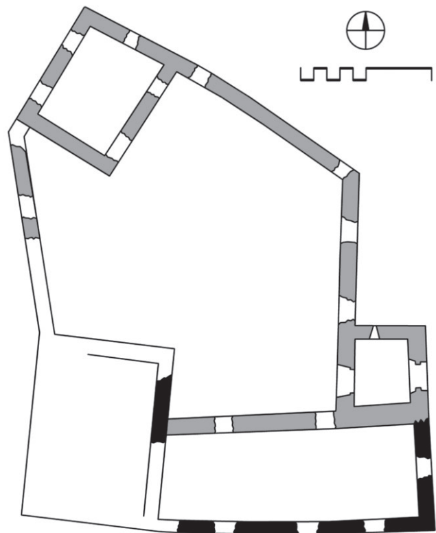
Thürn, romanische und frühgotische Bauphasen, schwarz: ältere Teile
