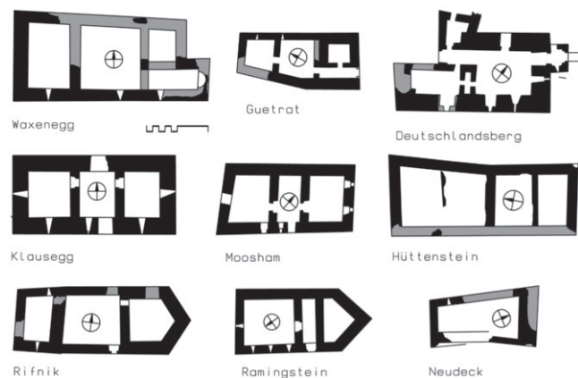
Zusammenstellung von charakteristischen Haus-Burgen um 1300
