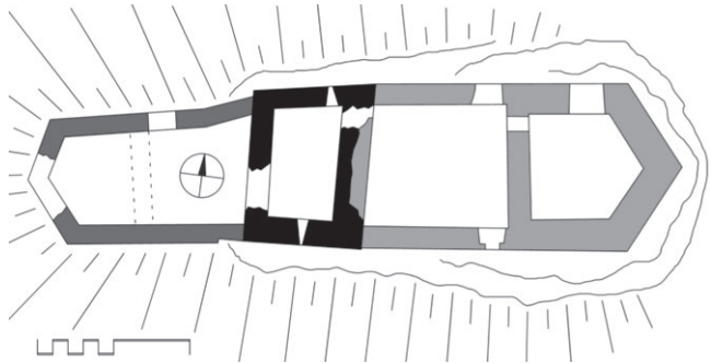
Reichenegg/Rifnik, Kernburg, schwarz: älterer Turm
