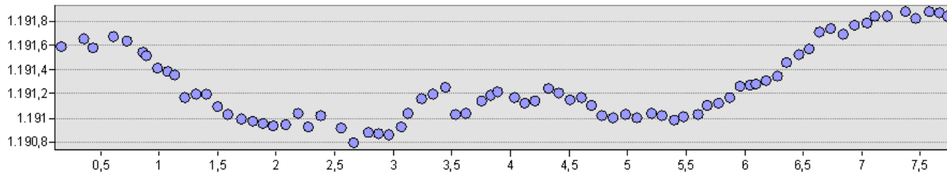
Profildigramm-Unterteil
